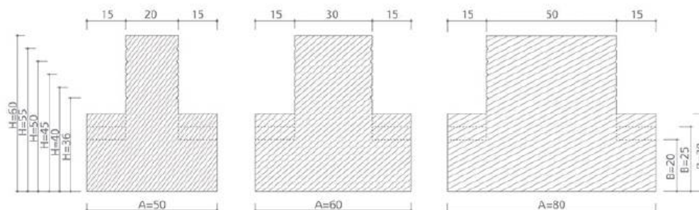
JÁCENAS SERIE JP - DIMENSIONES
