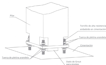
DETALLE DE FIJACIÓN ATORNILLADA
