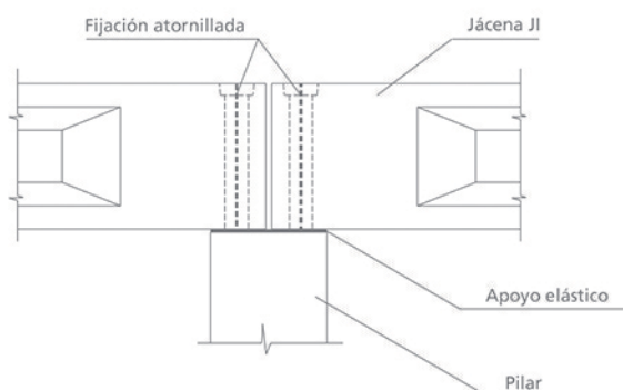
APOYO CENTRAL
