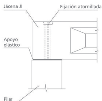
APOYO LATERAL
